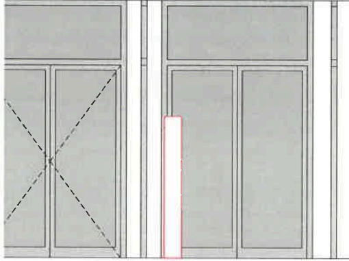
BOČNÍ POHLED
