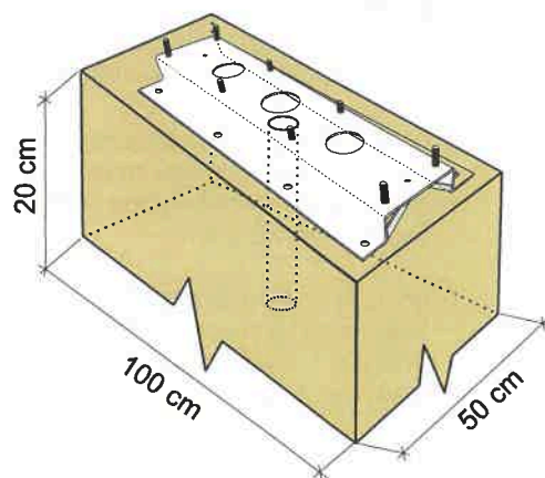
minimální rozměry betonového lůžka
